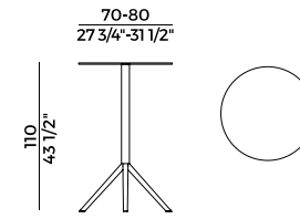
887/TAC tavolo pieghevole e impilabile \ folding and stackable table
