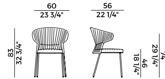
923/P-IMP poltroncina impilabile \ stackable small armchair ☞ ×4 con cuscino \ with cushion ☞ ×6 senza cuscino \ without cushion
