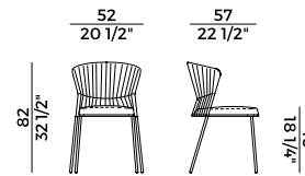
923 sedia impilabile \ stackable chair ☞ ×4 con cuscino \ with cushion ☞ ×6 senza cuscino \ without cushion
