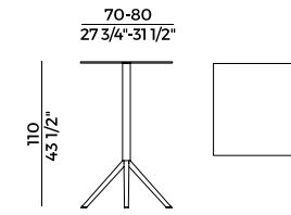
887/TAQ tavolo pieghevole e impilabile \ folding and stackable table
